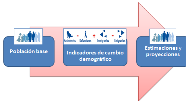
Figura 2 Método de componentes demográficos
